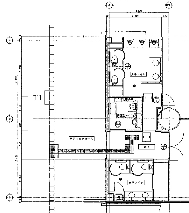
【改修後】建具キープラン S=1:50
