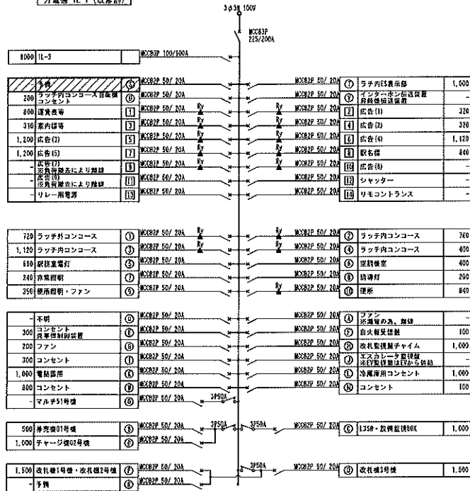
分電盤 1L-1 (改修前)
