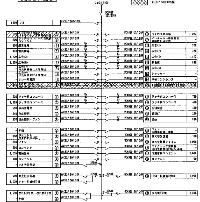
分電盤 1L-1 (改修後)
