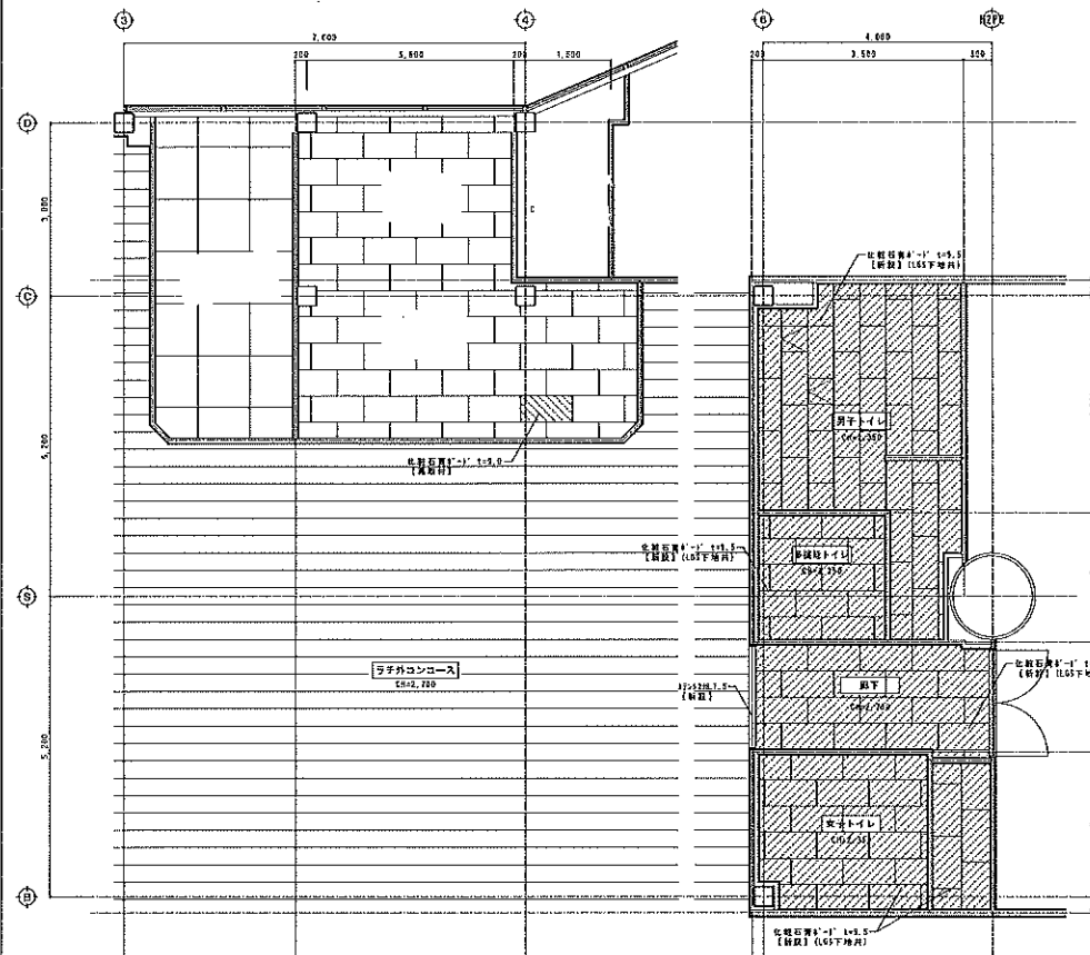
【改修後】天井伏図 S=1:50
