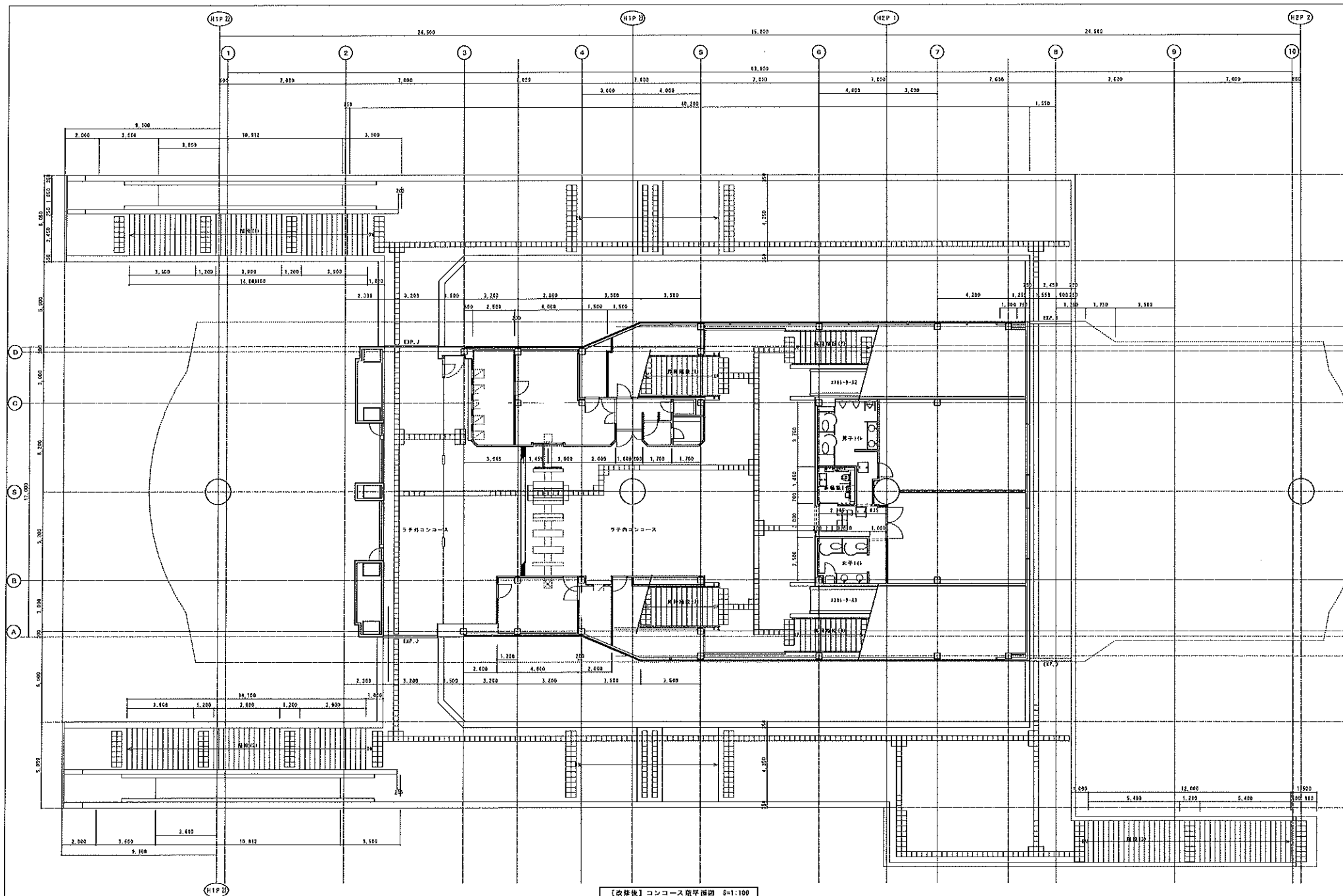
【改修後】コンコース階平面図 S=1:100
