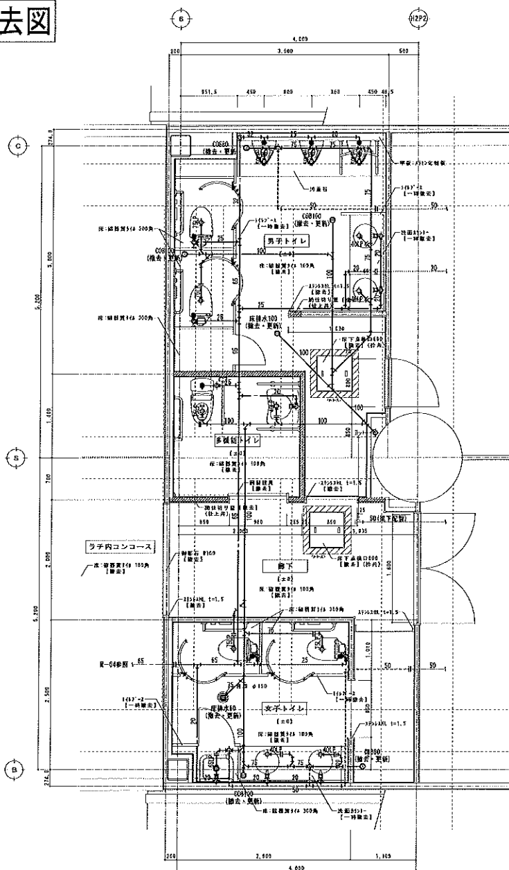
【改修前】平面詳細図 S=1:30
