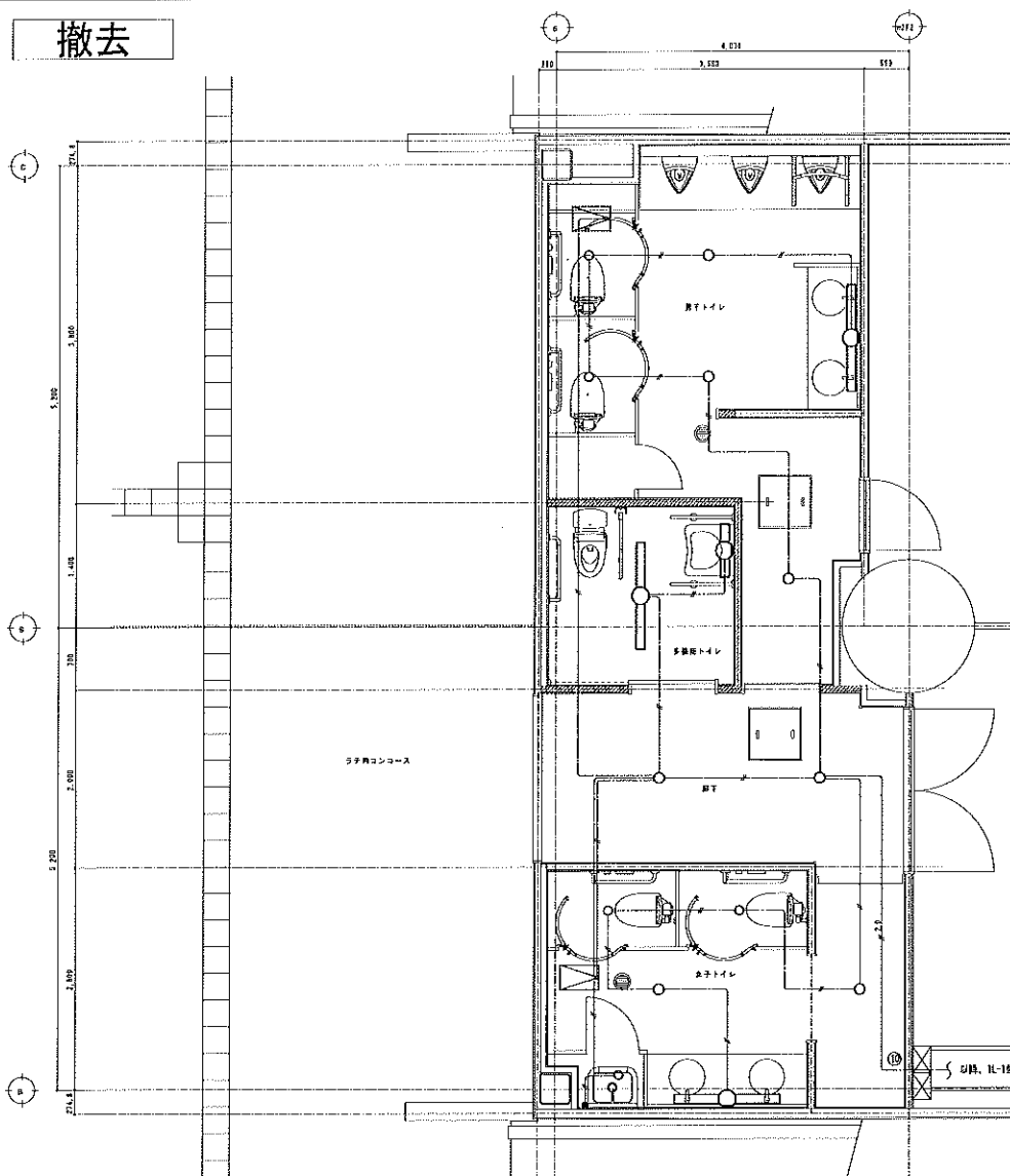
トイレ平面詳細図 S-1/30(撤去)
