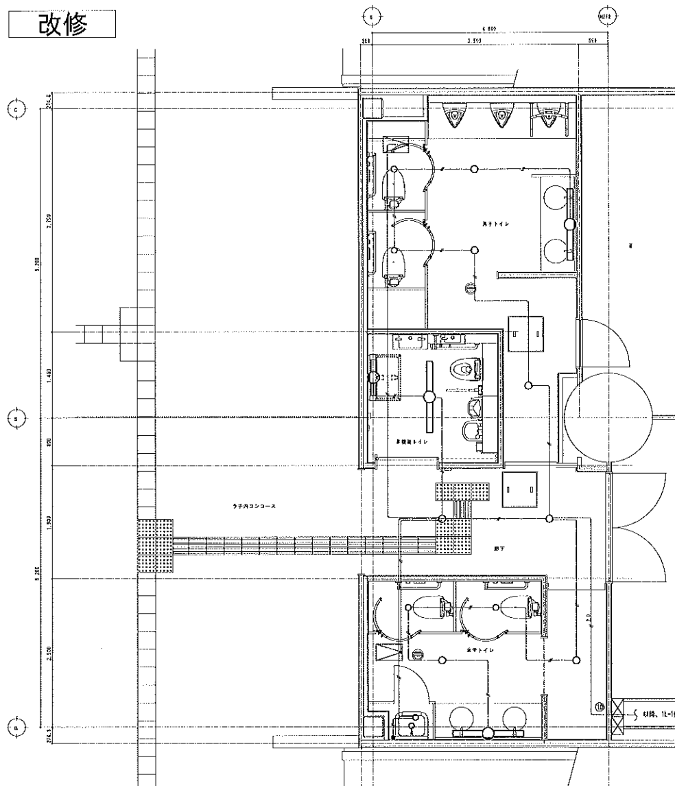
トイレ平面詳細図 S-1/30(改修)
