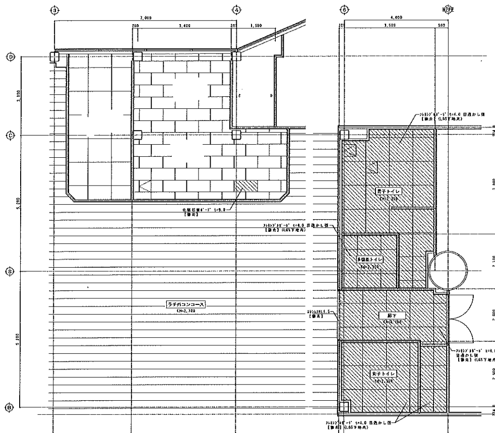
【改修前】天井伏図 S=1:50
