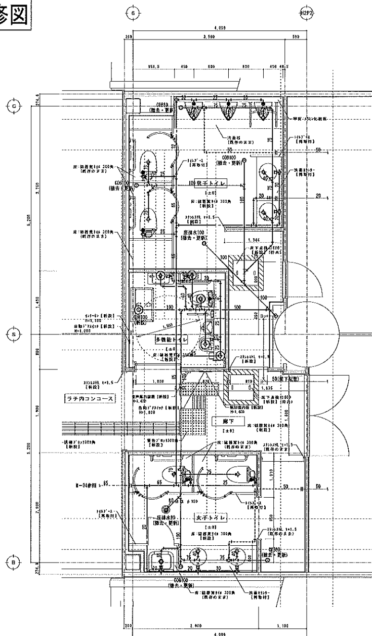
【改修後】平面詳細図 S=1:30
