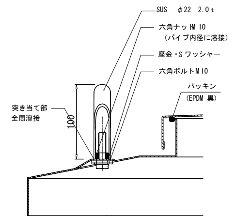
A-A 断面矢示図 (尺度=1:2)
