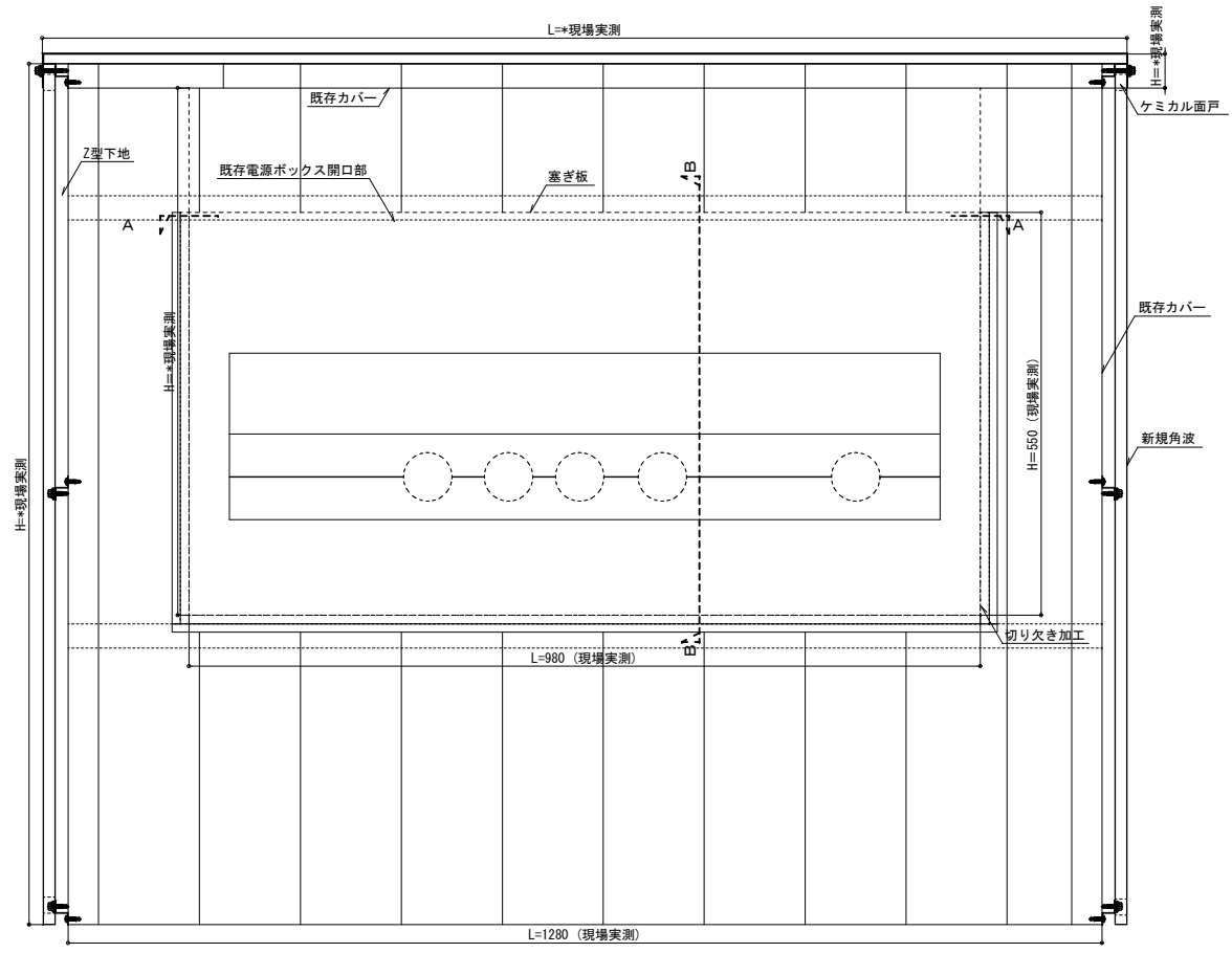
立面図 1 S=1:5
