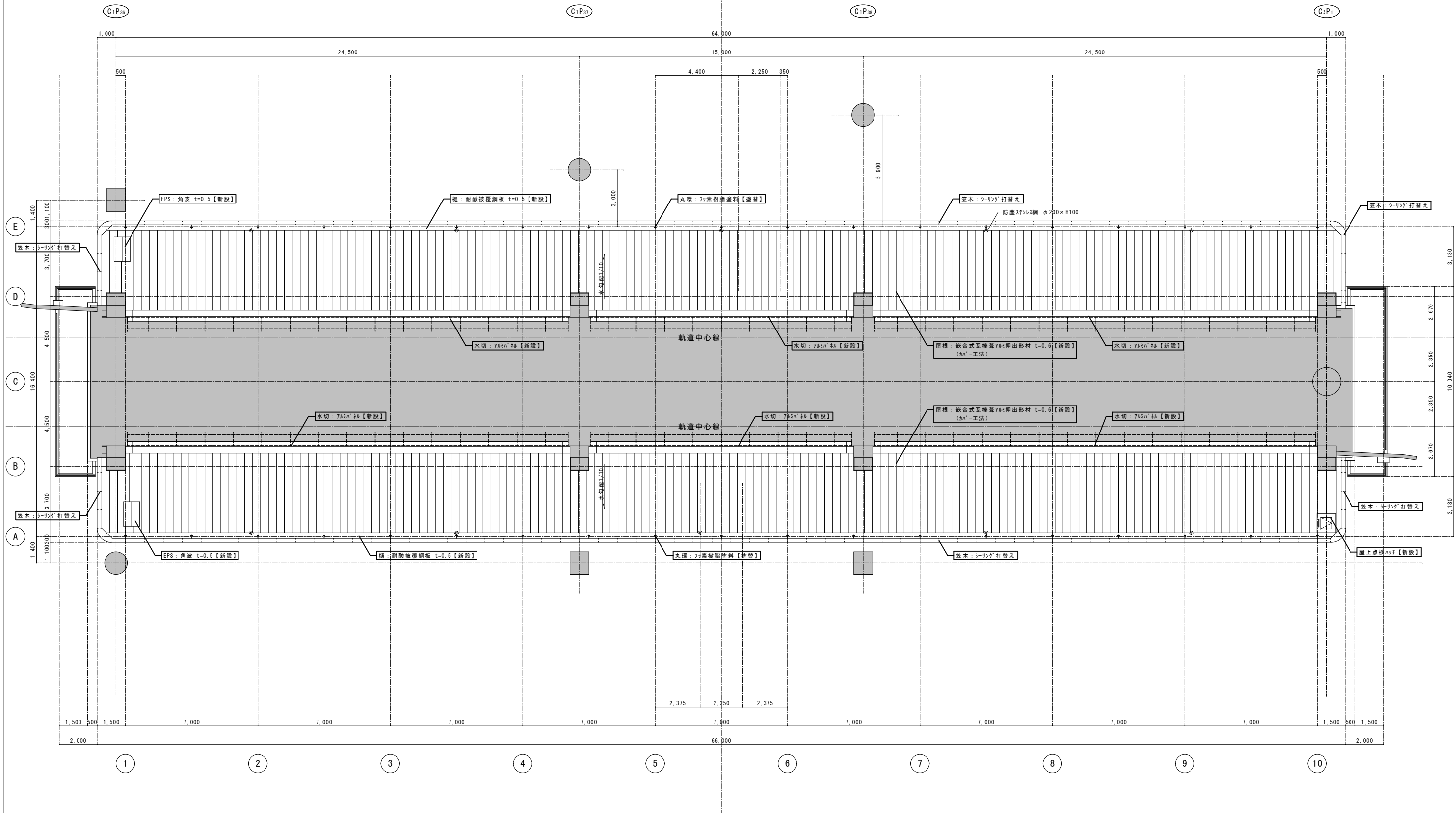
【改修後】屋根伏図 S=1:100
