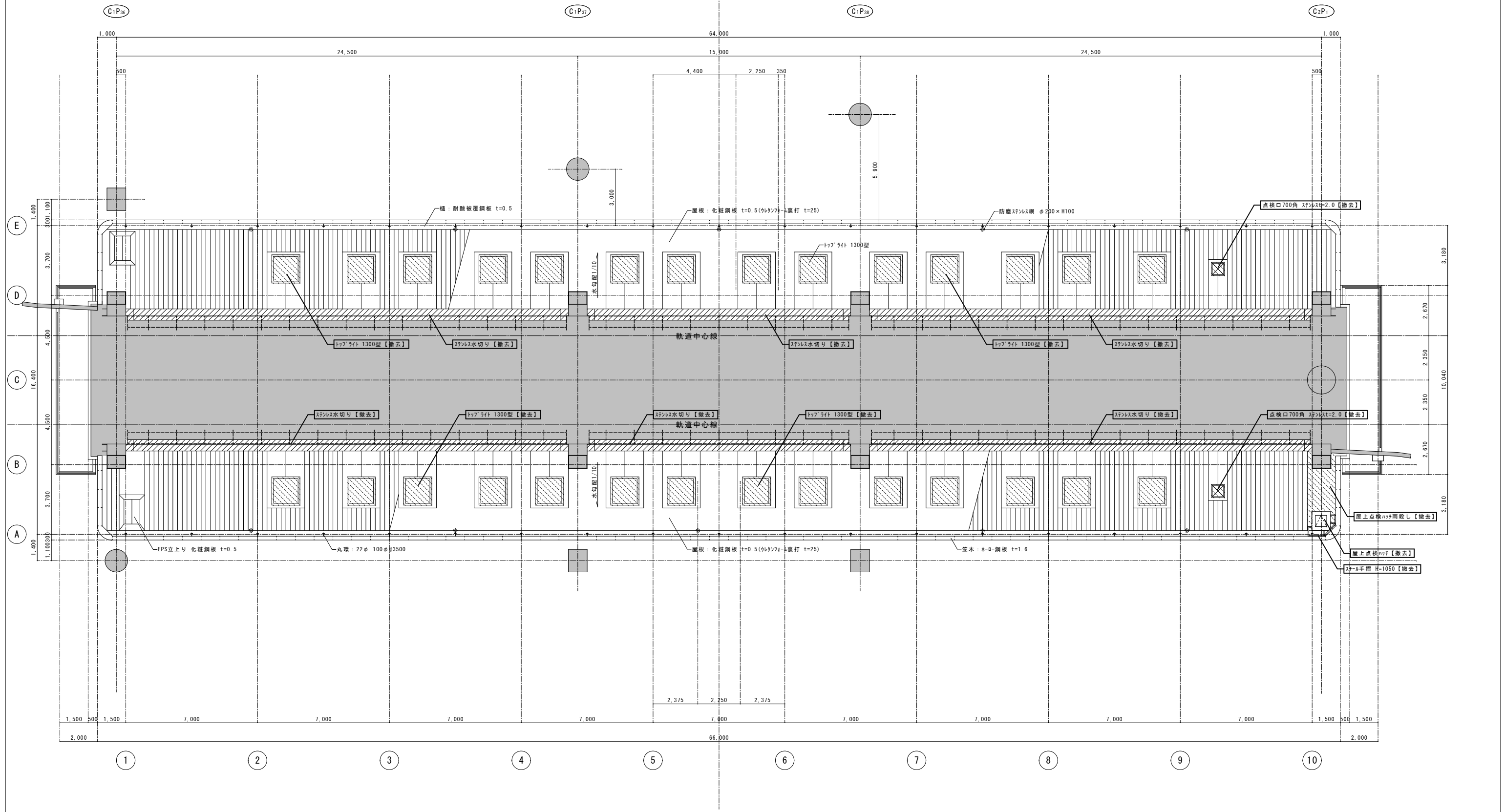
【改修前】屋根伏図 S=1:100
