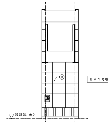
南側立面図 S=1:100
