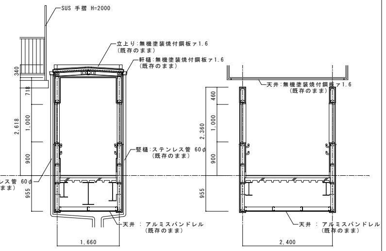
断面詳細図 S=1:50
