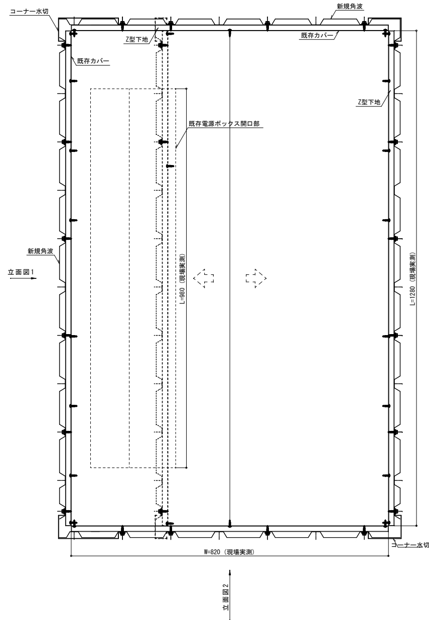
EPS 平面図 S=1:5
