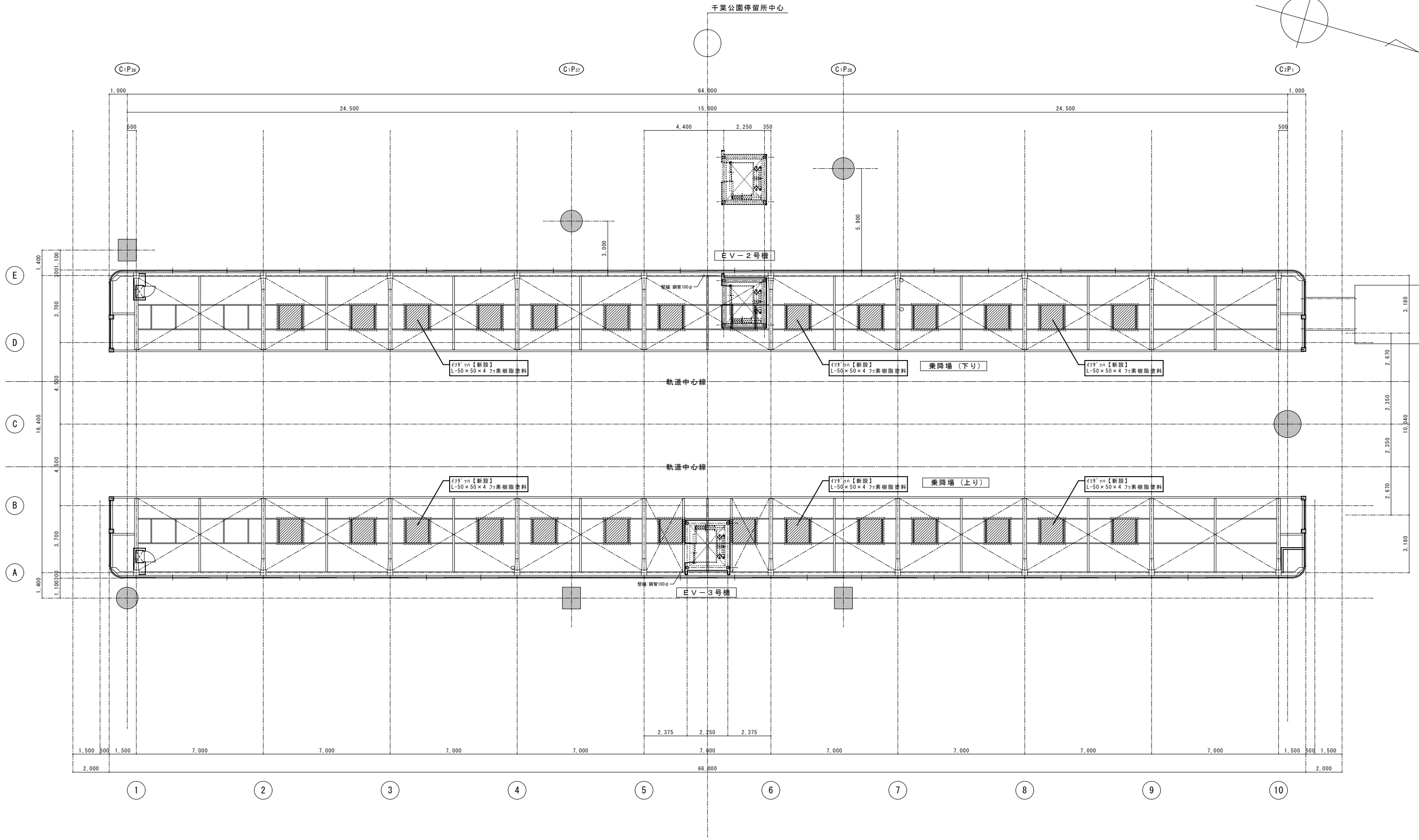
乗降場階 天井伏図 S=1:100
