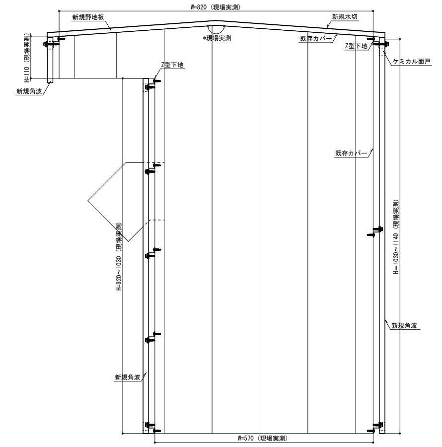
立面図 2 S=1:5
