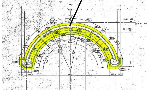
A 矢視図
