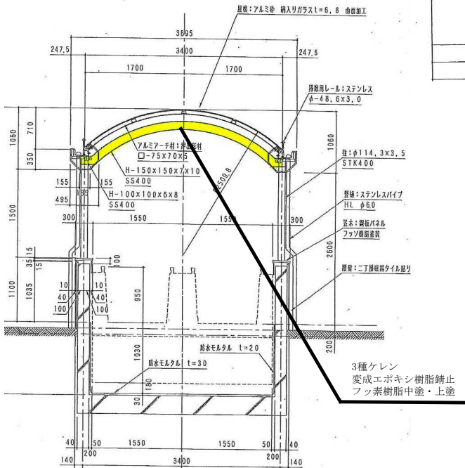
外エスカレーター横断面詳細図
