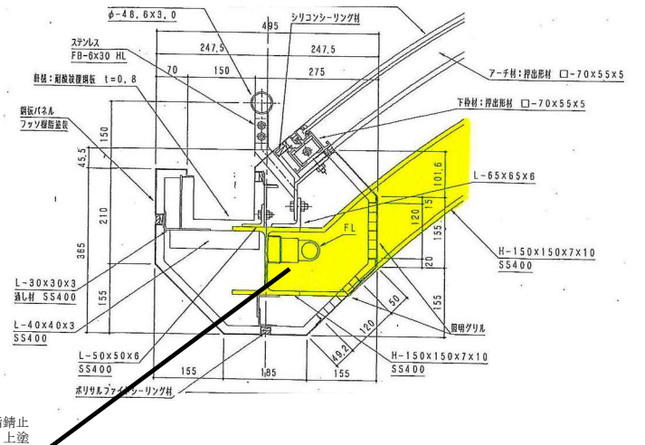
雨樋詳細図
