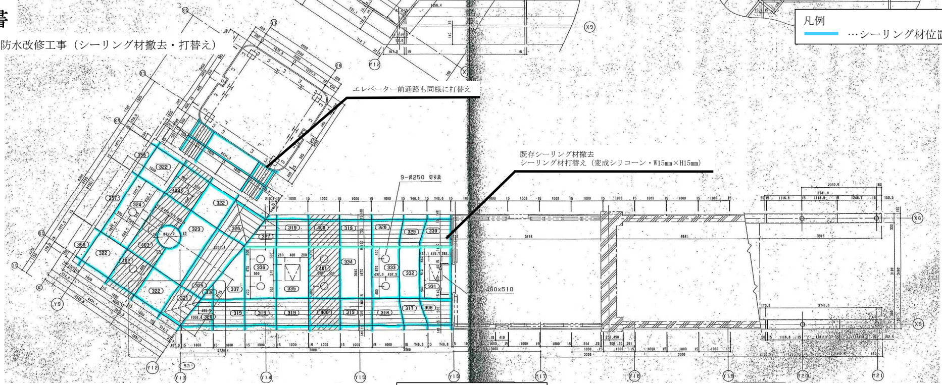
外エスカレーター軒天井図
