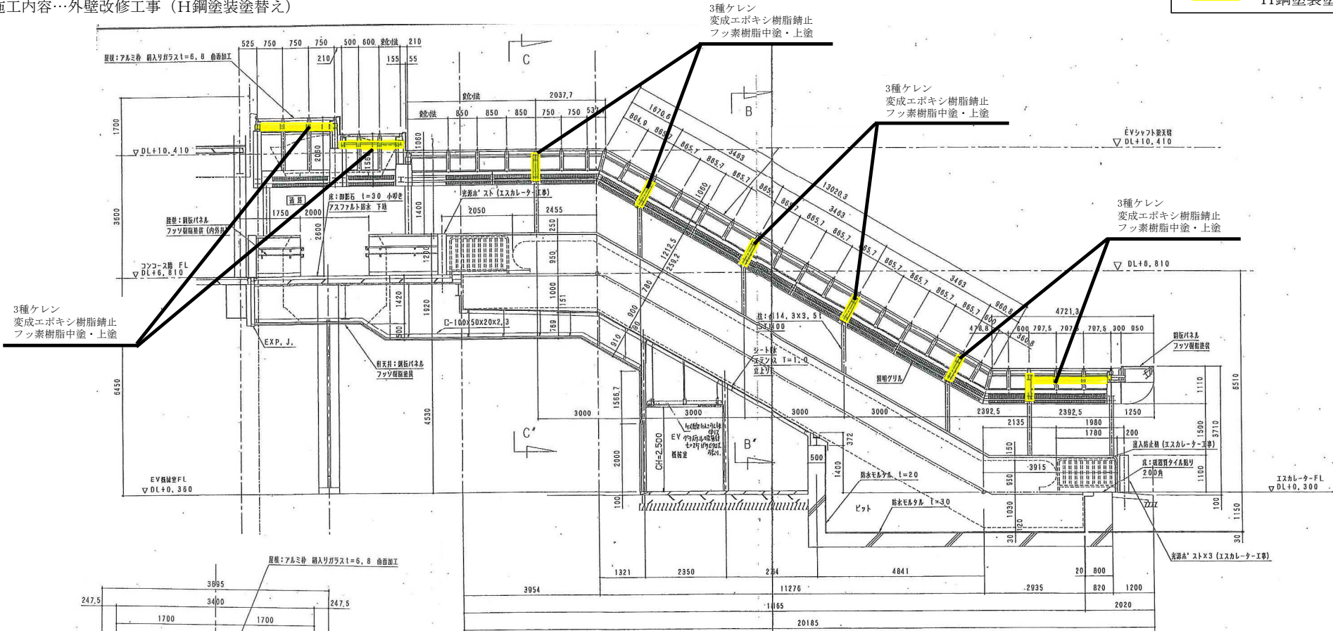
外エスカレーター縦断面詳細図
