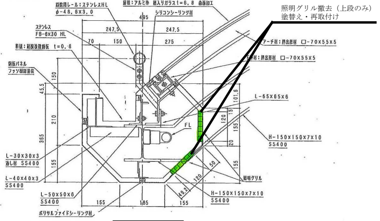
雨樋詳細図
