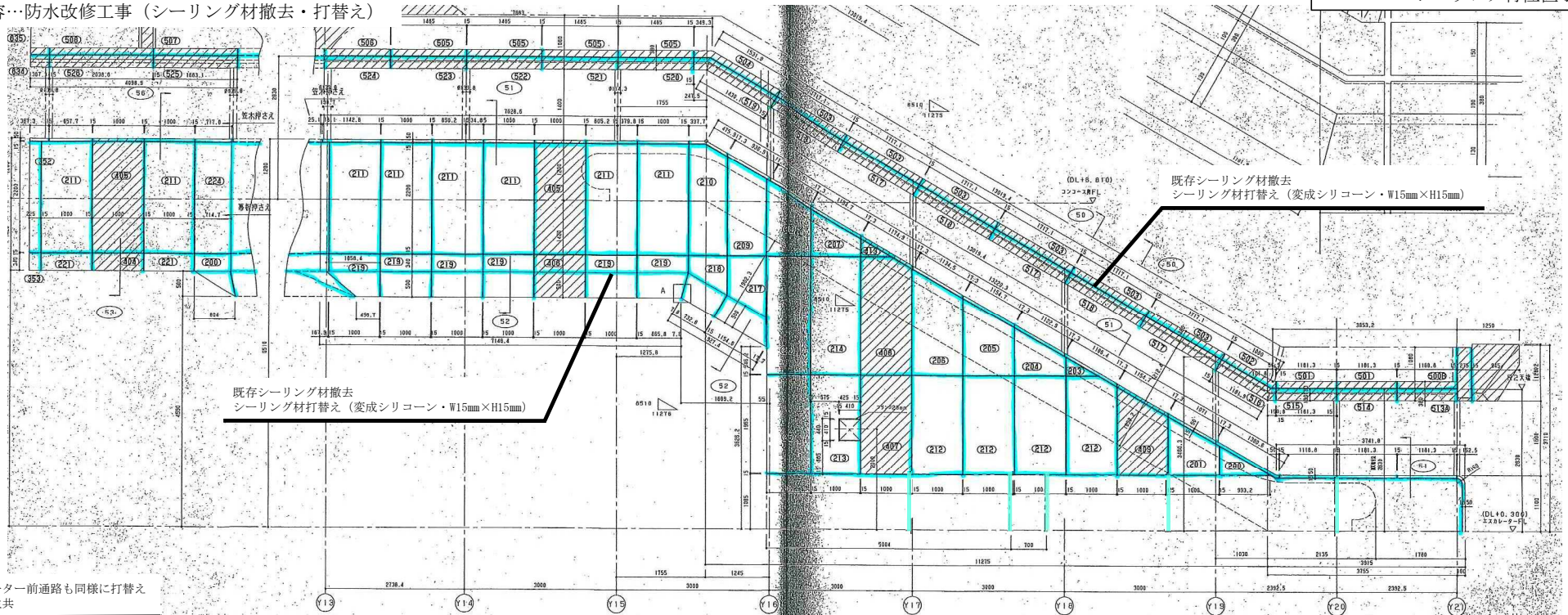
外エスカレーター北立面図
