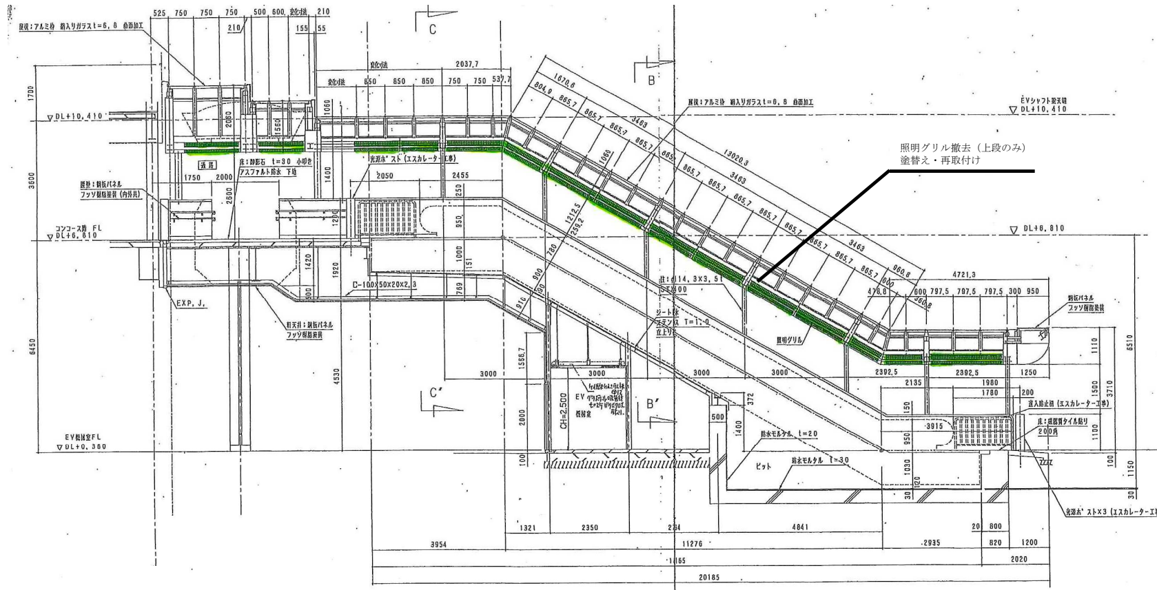
外エスカレーター縦断面詳細図
