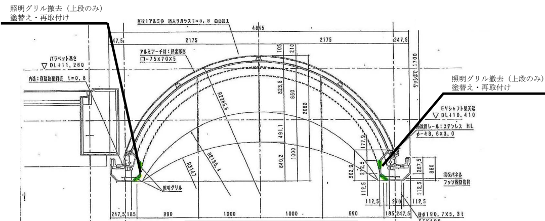
外エスカレーター横断面詳細図
