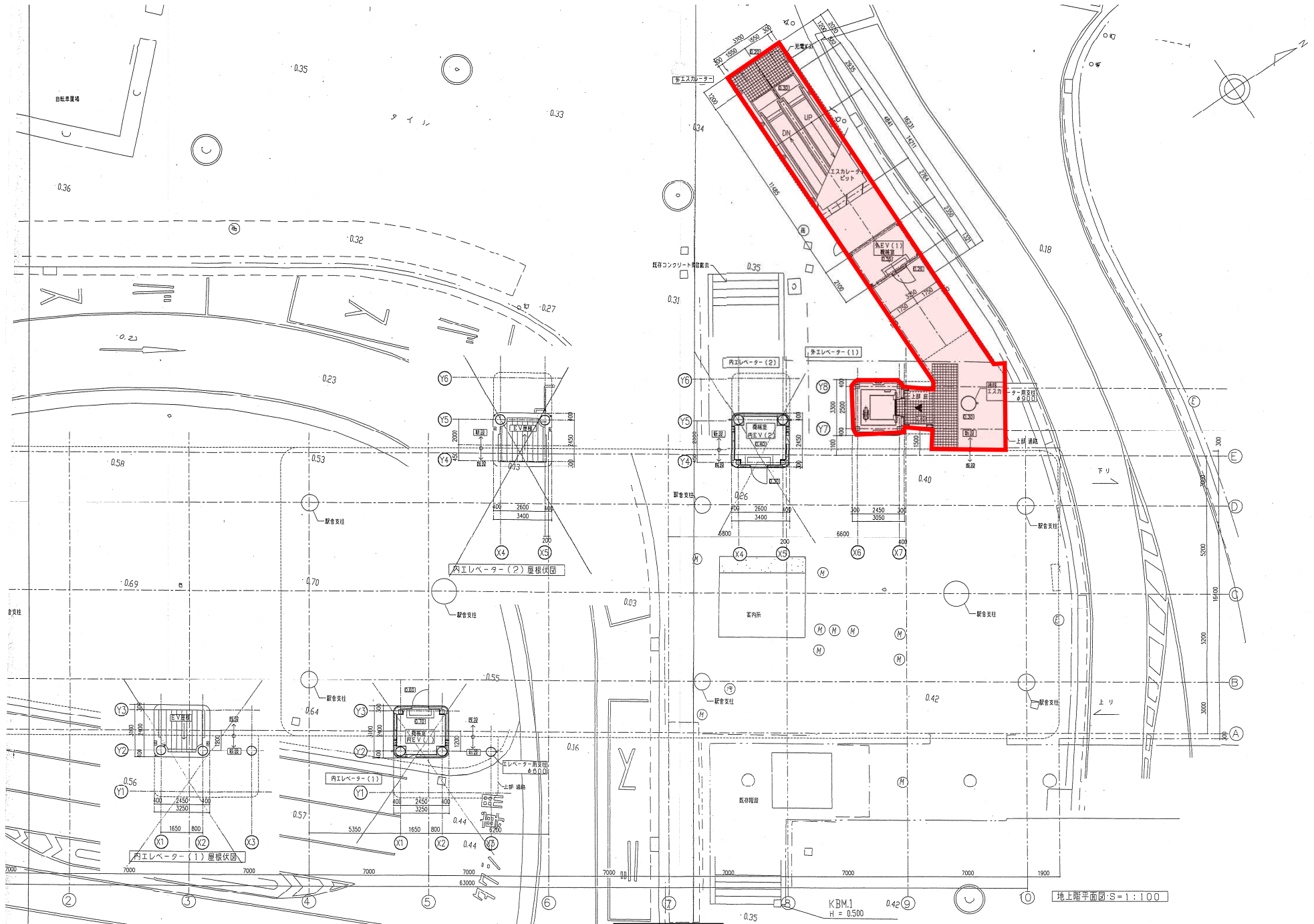
地上階平面図
