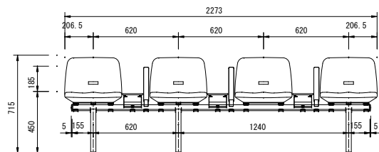
<桁式>
