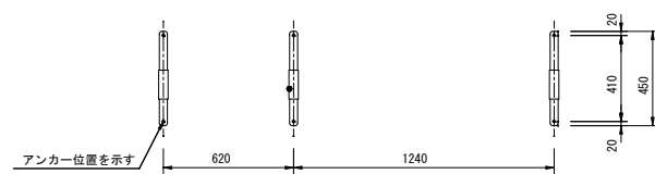
アンカー伏図 S=1/20
