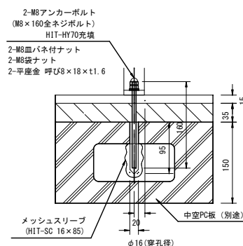
床取付詳細図 S=1/5
