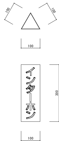
⑪ インターホン (サイン) W100×H300mm 三角柱
