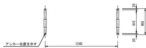
アンカー伏図 S=1/20
