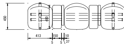
アンカー伏図 S=1/20
