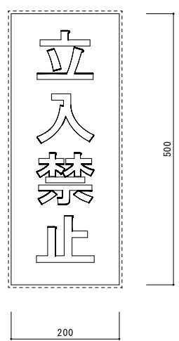
⑭ 軌道内立入禁止 (サイン) W200×H500mm (下地サイズ W210×H510mm) (別途工事)
