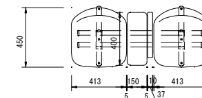
アンカー伏図 S=1/20
