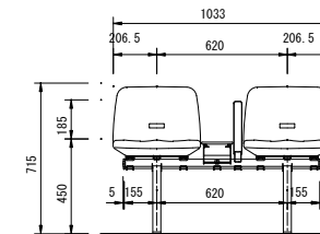
<桁式>
