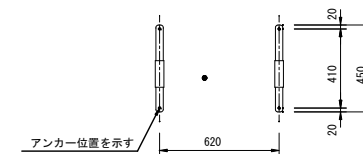
アンカー伏図 S=1/20
