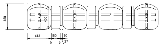
アンカー伏図 S=1/20
