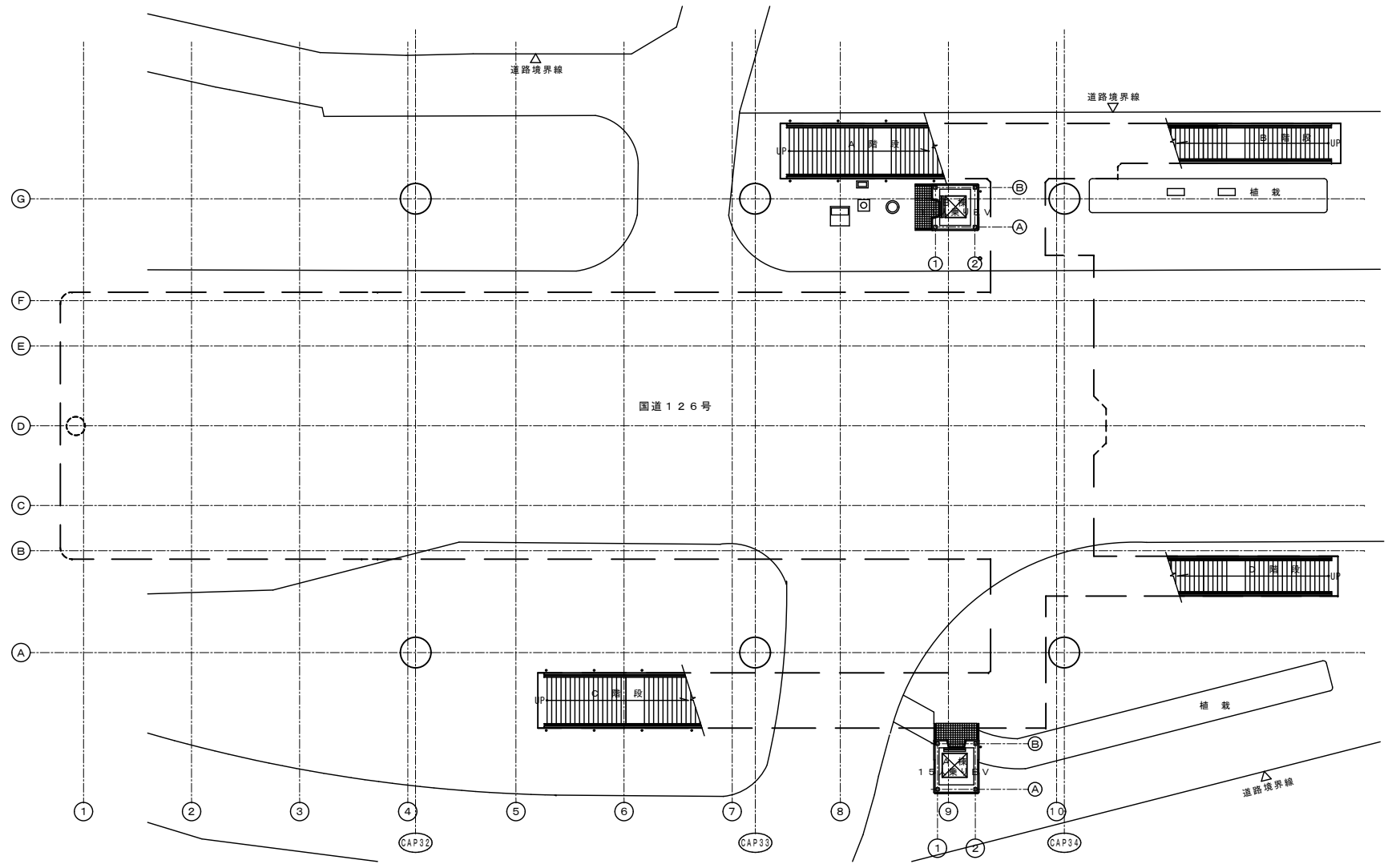
配置図 S=1:200
