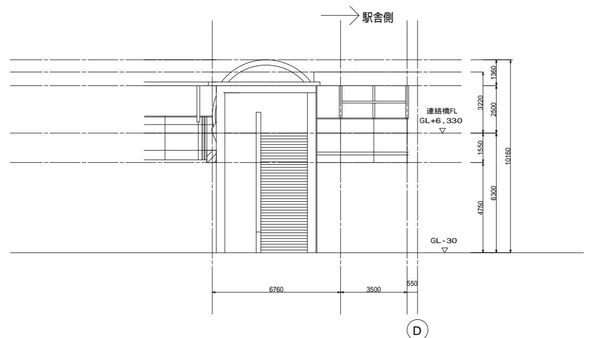
北自由通路 西立面図 (S:1/200)
