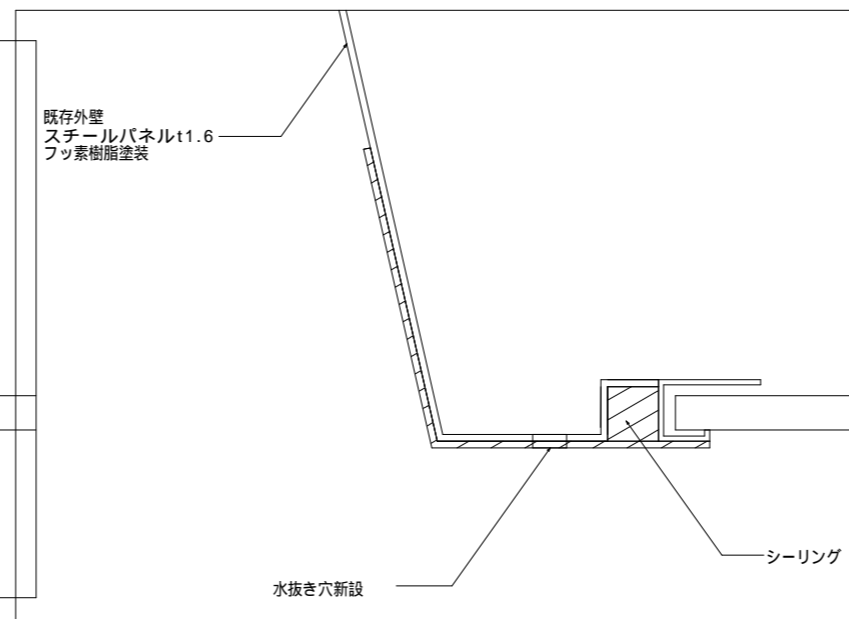
自由通路階段 外壁補修部詳細図 (S:1/2)
