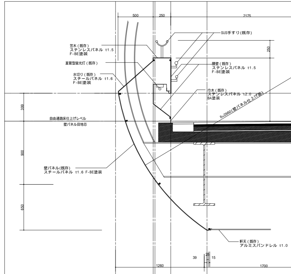
壁断面形状A 詳細図 (S:1/30)
