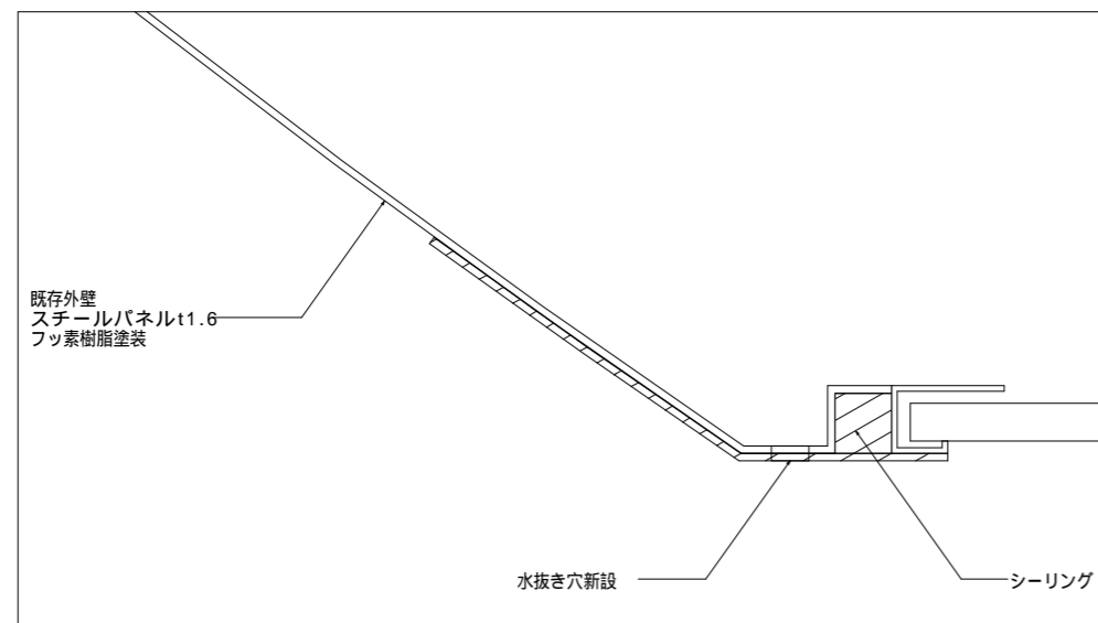
自由通路 外壁補修部詳細図 (S:1/2)
