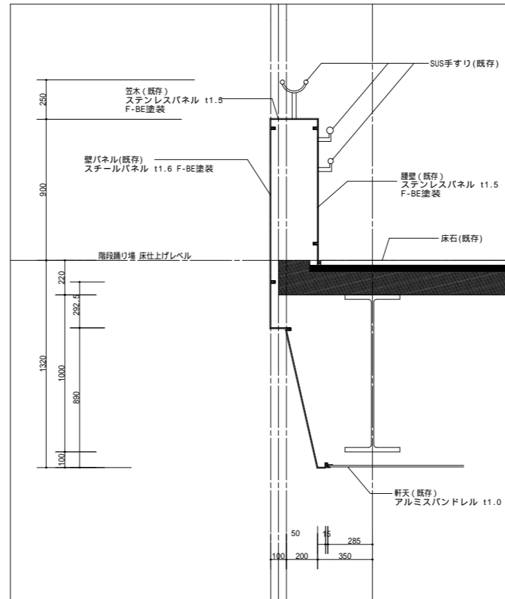
壁断面形状B 詳細図 (S:1/30)
