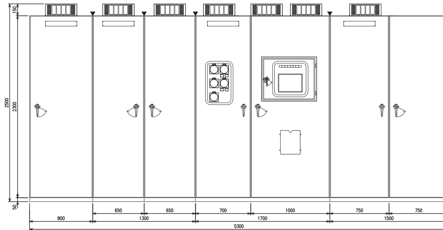
正面図
