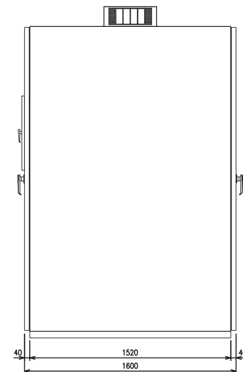
側面図
