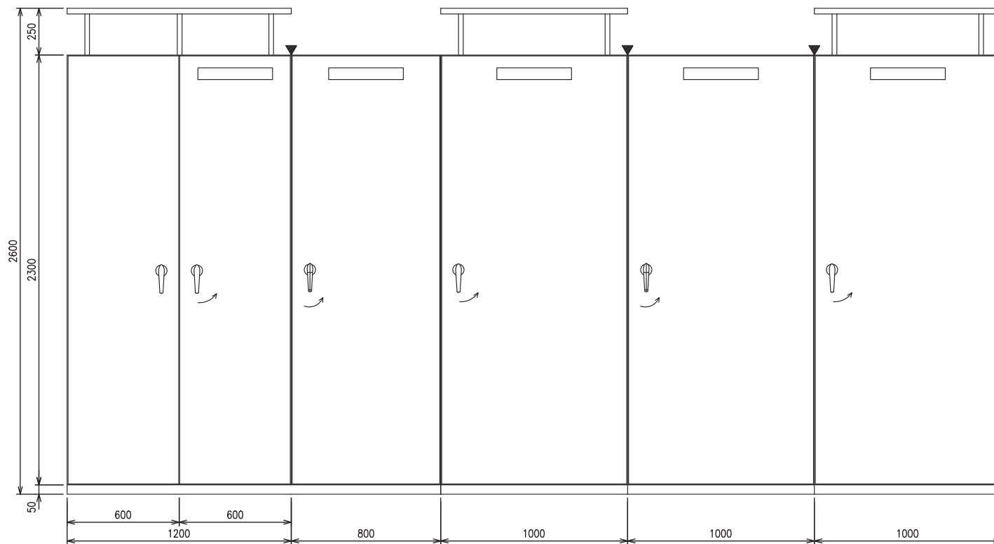
正面図
