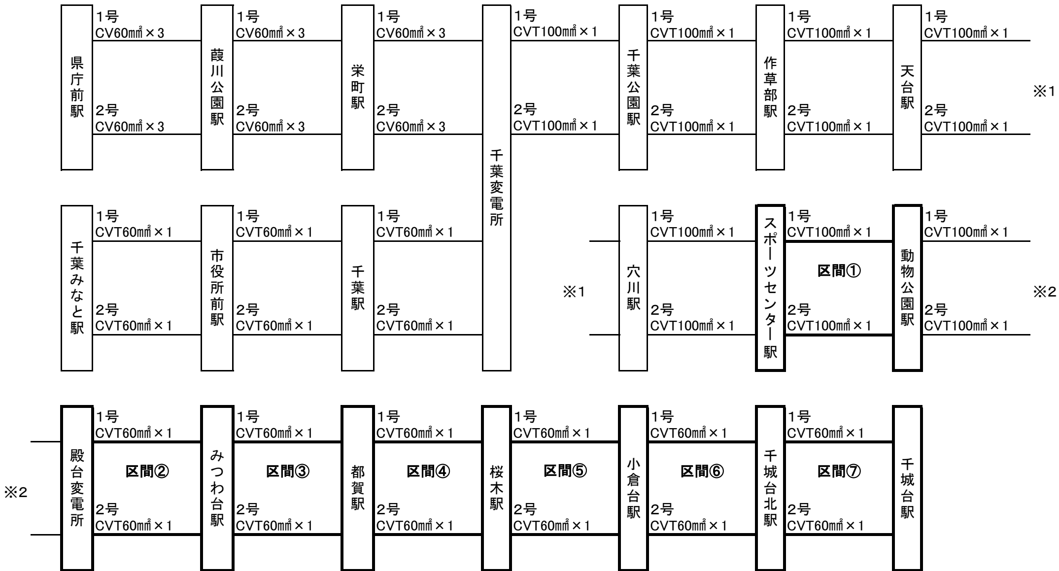
別図1 変電所および各駅配電系統図(既設)
