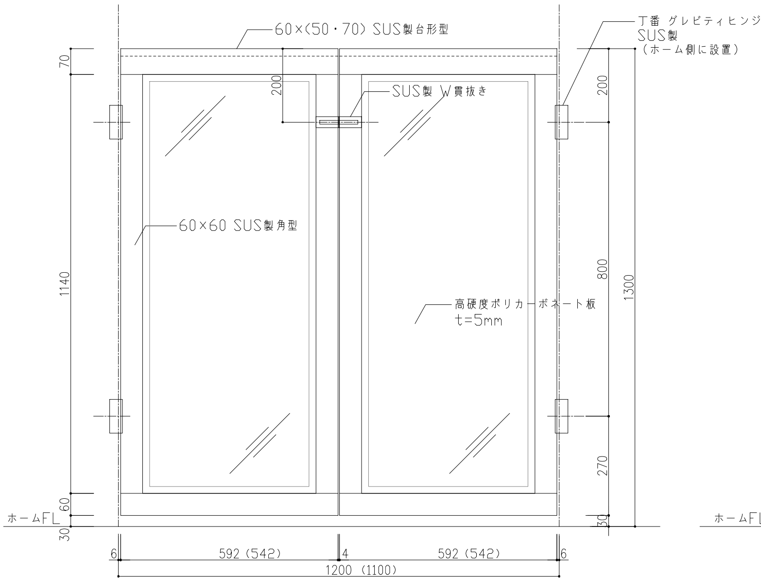
フレーム：角材仕様 （軌道側姿図）
