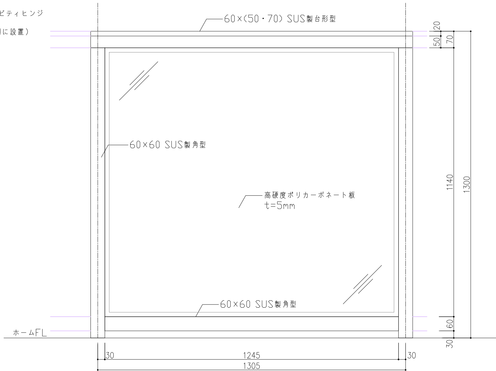
フレーム、支柱：角材仕様 （ホーム側姿図）
